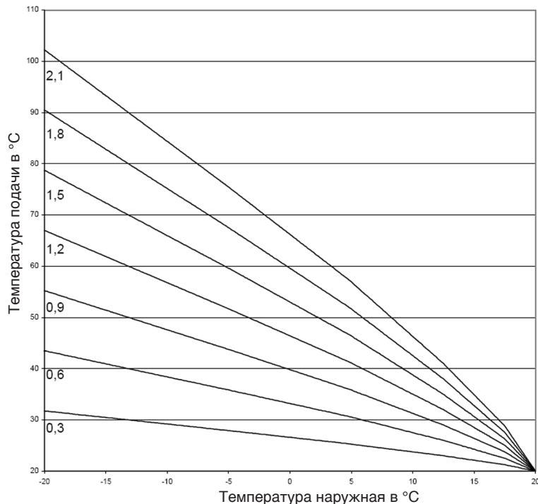
Кривые нагрева
