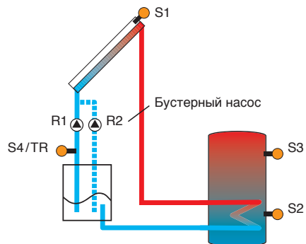
Примерная схема установки обратного дренирования (R2 = бустерный насос)
