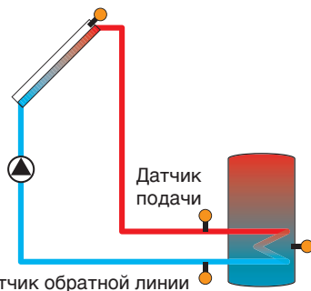
Пример расположения датчиков подачи и обраты
