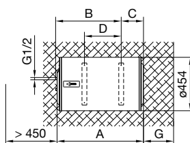
Sl. 2: Horizontalno postavljanje na zid
