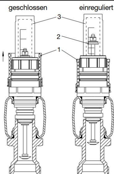
Рис. 7.2 Настройка ротаметров (1 – 4 л/мин)
