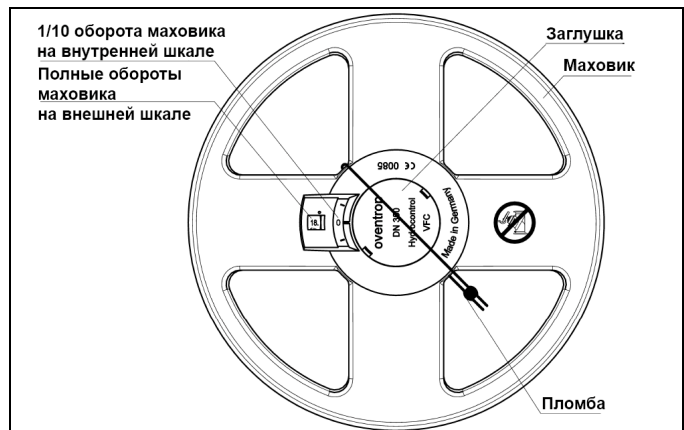
Рис. 7.1 Настройка
