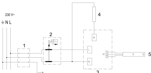
Рис. 5: Електрична схема
