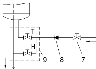
Малюнок 3: Безнагрірна (відкрита) система
