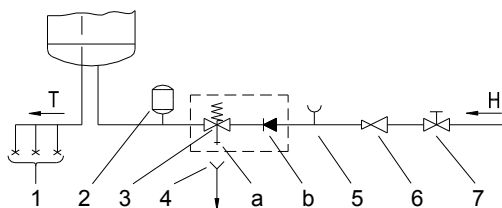
Малюнок 2: Нагрірна (закрита) система
