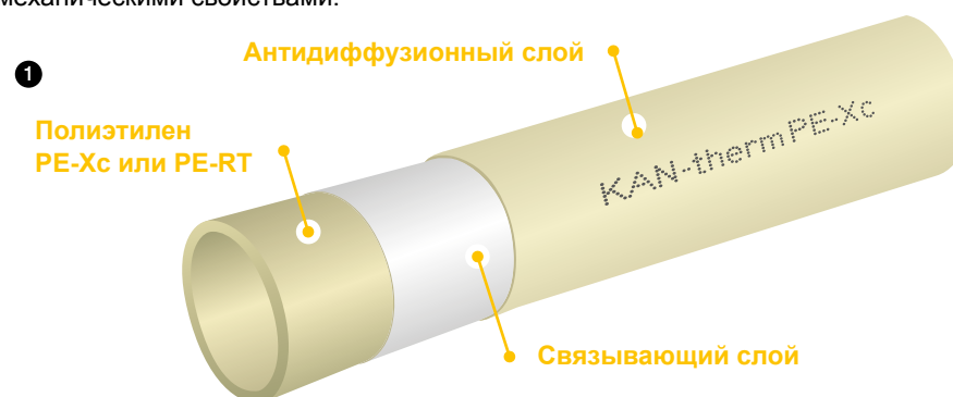
1. Конструкция трубы PE-Xc и PE-RT.
