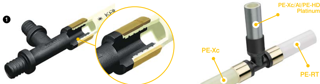
1. Соединение Push в разрезе.
